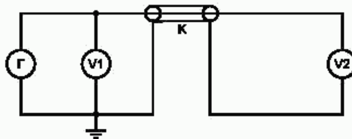
Г — генератор; V1, V2 — вольтметры; К — кабель
