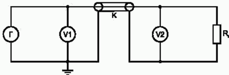
Г — генератор; V1, V2 — вольтметры; К — кабель; Rн — нагрузочное сопротивление
